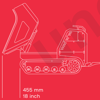
→ Provedení s otočnou korbou
